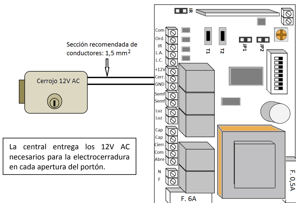
Esquema 1- Conexión de Electrocerradura
