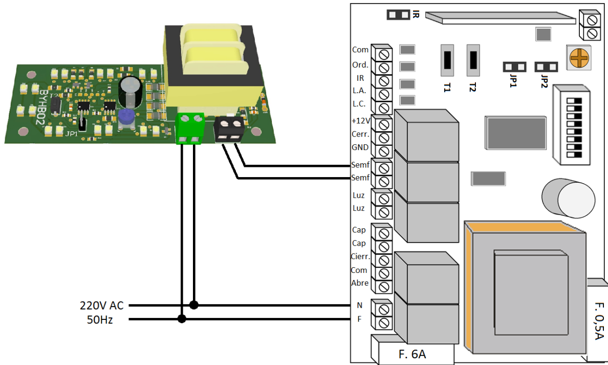
Esquema 4 - Conexión de Baliza 4 Cables
